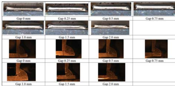
Figura 3. Fotografías y macrografías de soldadura de variación de gap en relación a los parámetros elegidos.
