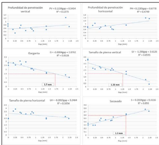
Figura 4. Gráficas de correlación lineal de tamaño de gap en relación a las diferentes características medidas de calidad de la soldadura.
