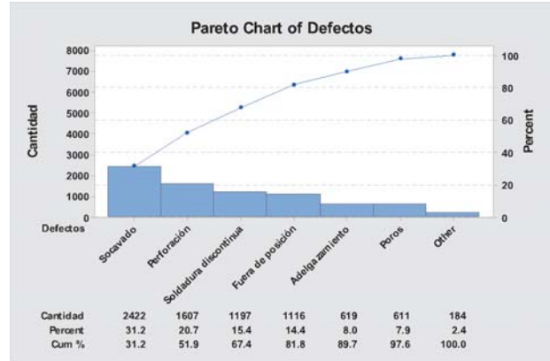
Figura 1. Diagrama de pareto de defectos de soldadura.
