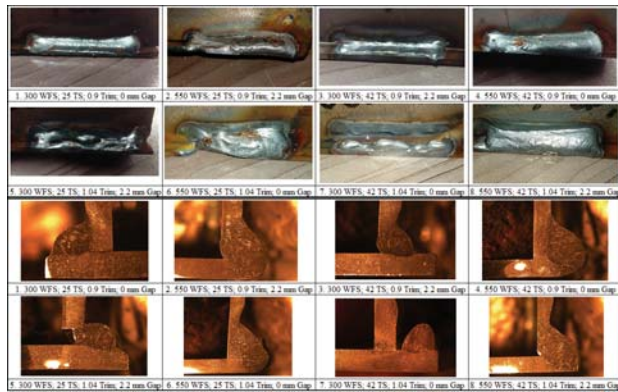
Figura 7. Fotografías y macrográficas de soldadura de las corridas del DFF
