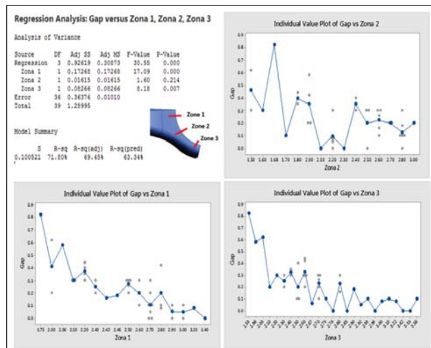
Figura 2. Análisis de varianzas en relación del trim de la superficie del estampado superior con respecto al gap.
